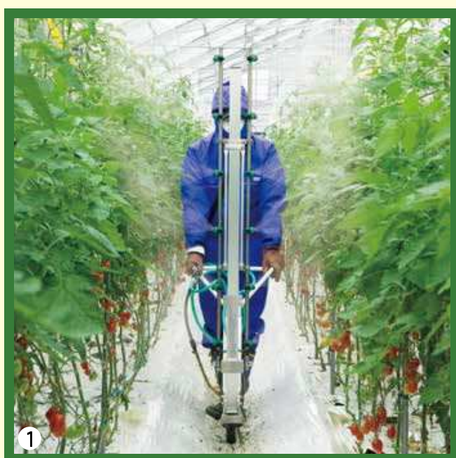
①カートジェッター GR 型 1 輪 散布例
